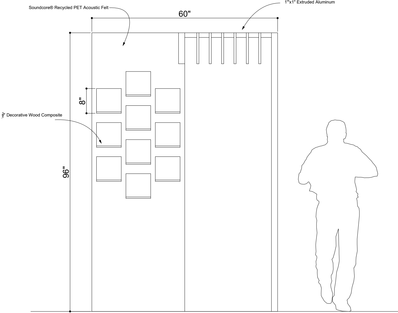
① ELEVATION 1
